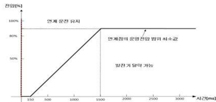
[순시전압저하시 연계운전 유지성능]
