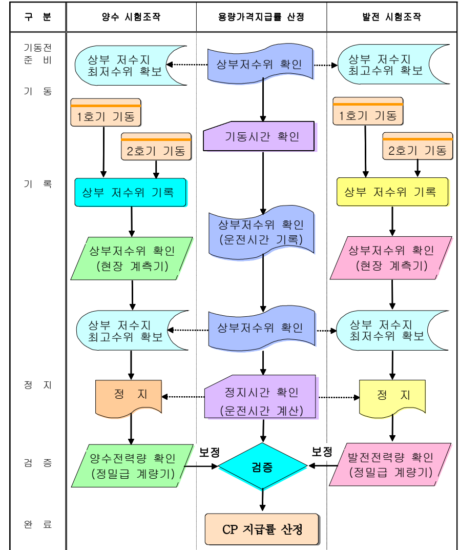
양수발전소 용량가격지급률 ( \xi_i ) 시험 흐름도
