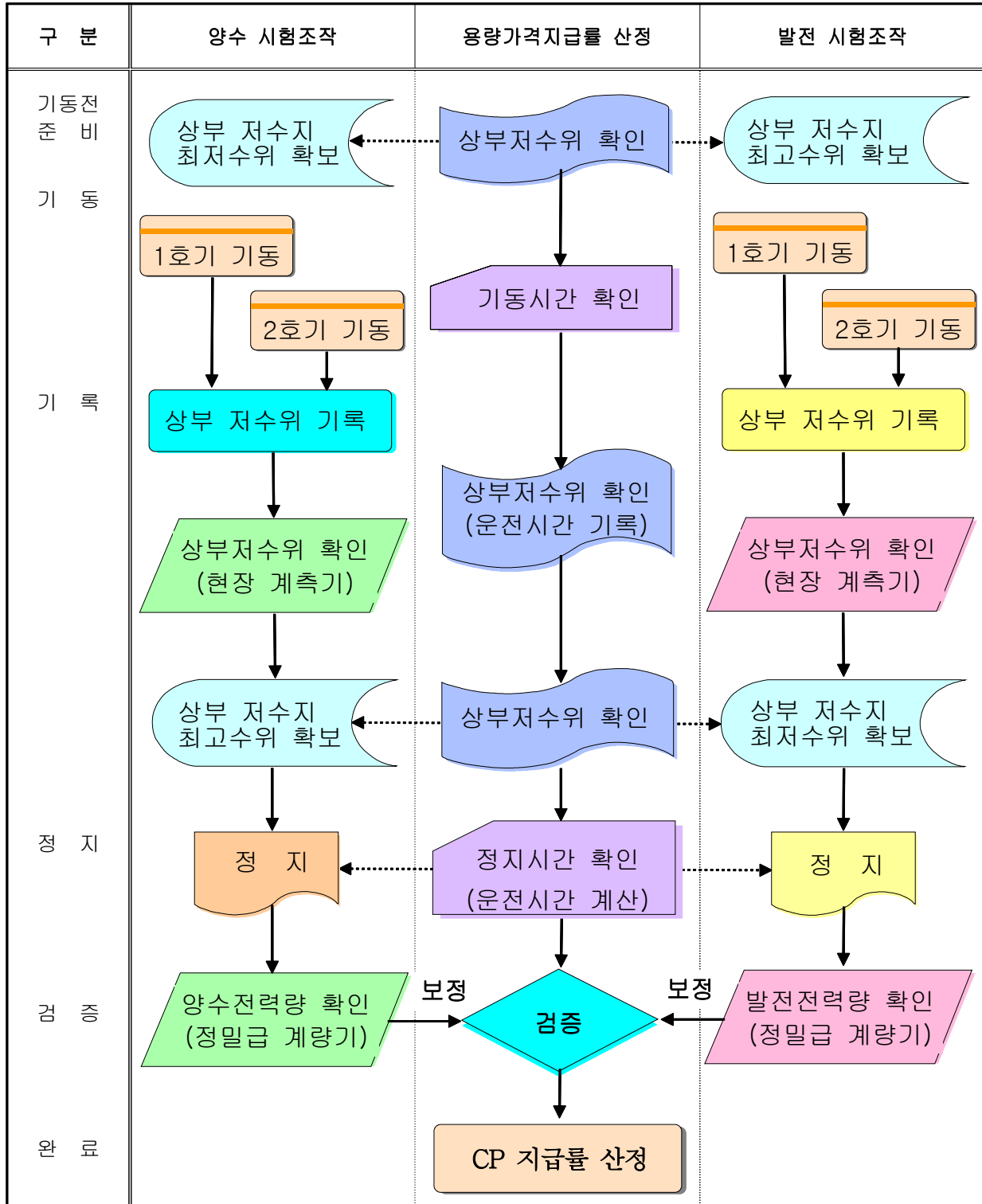
양수발전소 용량가격지급률( \xi_i ) 시험 흐름도
