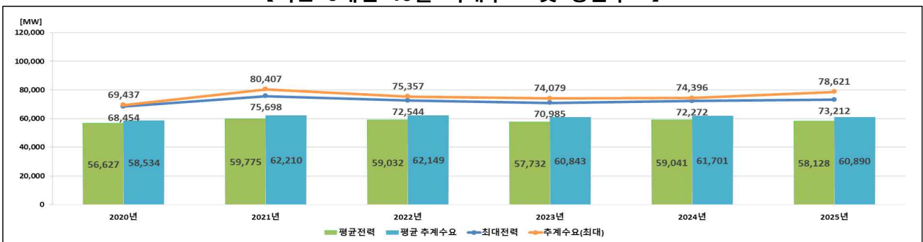
【최근 6개년 10월 최대수요 및 평균수요】
