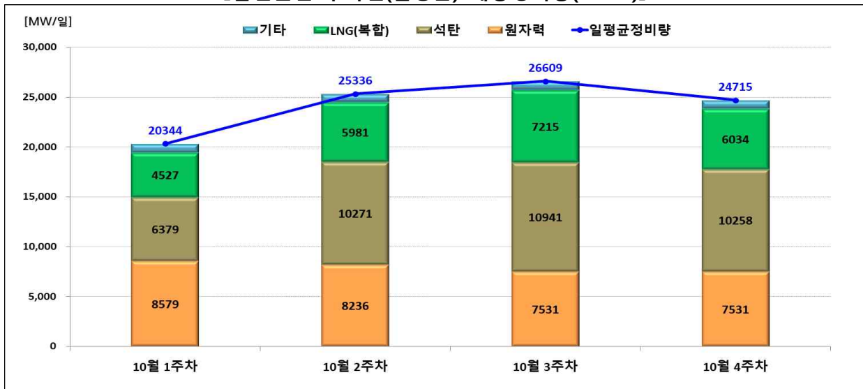
【발전원별 주차별(일평균) 예방정비량('25.10)】
