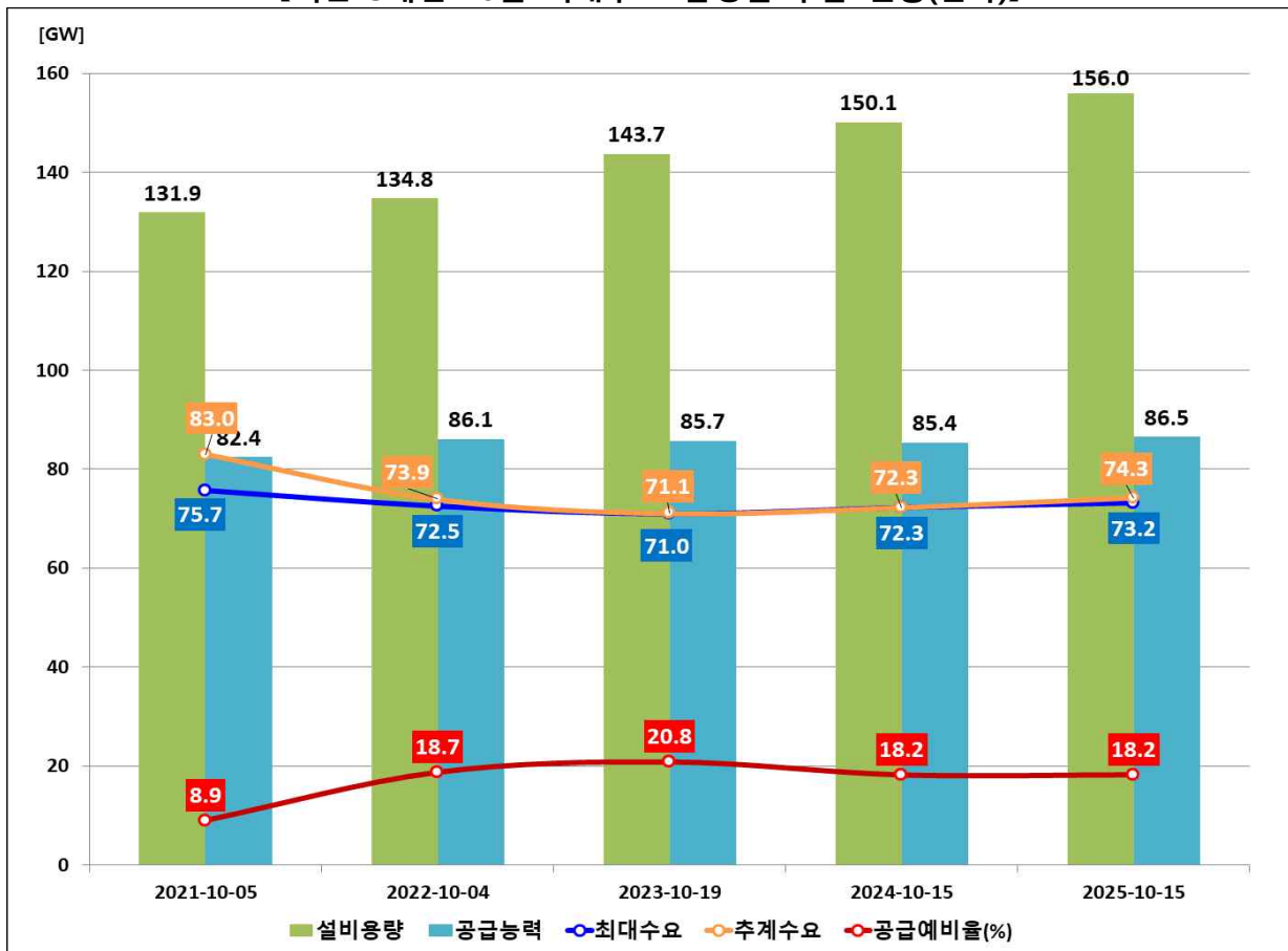
【최근 5개년 10월 최대수요 발생일 수급 현황(전국)】
