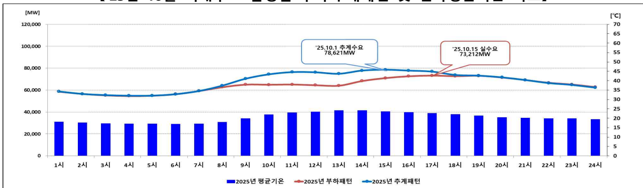
['25년 10월 최대수요 발생일 부하-추계패턴 및 전국평균기온 비교]
